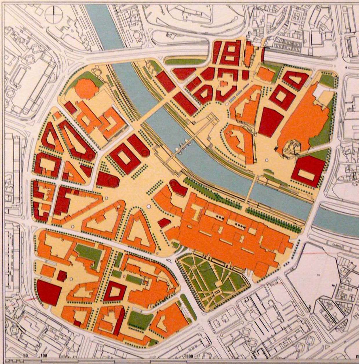
ДУП за Малиот ринг Скопје, Грчев, Коробар, М. Пенчиќ, 1997 год.
