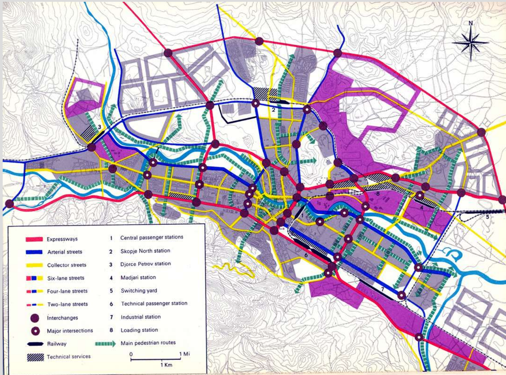
Скопје, планирана состојба на сообраќајната мрежа во 1981 год.
