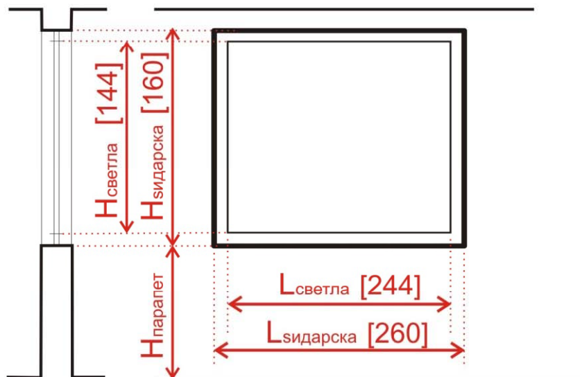
ОБЕЛЕЖУВАЊЕ НА ПРОЗОР
