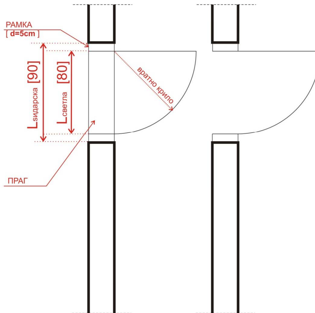
ОБЕЛЕЖУВАЊЕ НА ВНАТРЕШНА ВРАТА
