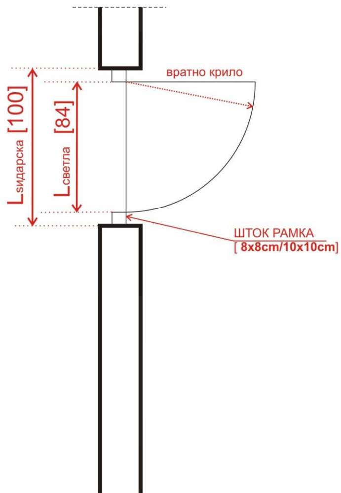
ОБЕЛЕЖУВАЊЕ НА НАДВОРЕШНА ВРАТА
