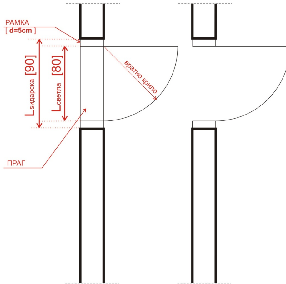
ОБЕЛЕЖУВАЊЕ НА ВНАТРЕШНА ВРАТА
