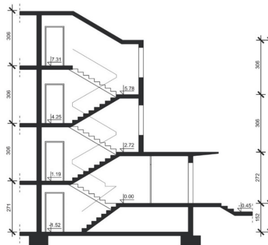
вертикален пресек
