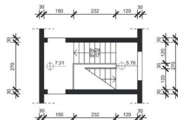
основа на последен кат
