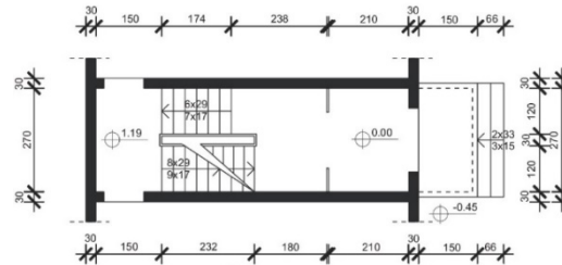
основа на приземје
