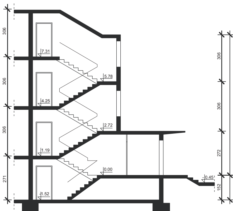
вертикален пресек
