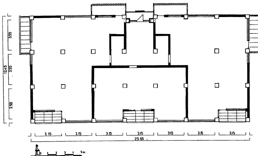
OSNOVA NA I VI KAT
