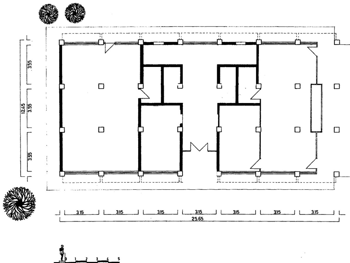
OSNOVA NA PRIZEMJE
