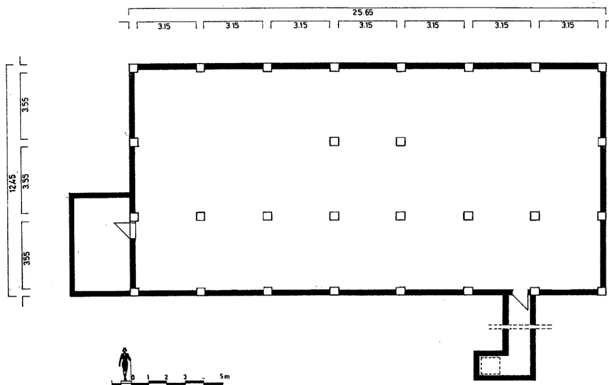
OSNOVA NA PODRUM
